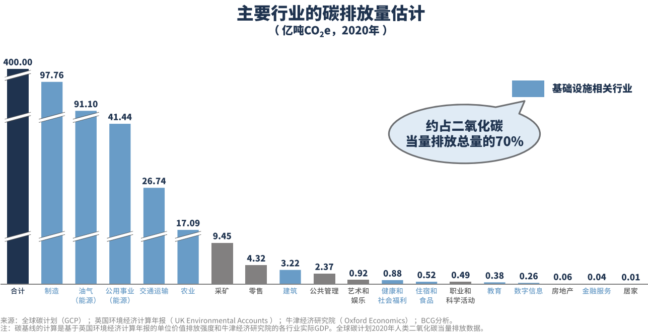
图 5. 基础设施相关行业贡献了约全球温室气体总排放量的 70%，值得特别关注
